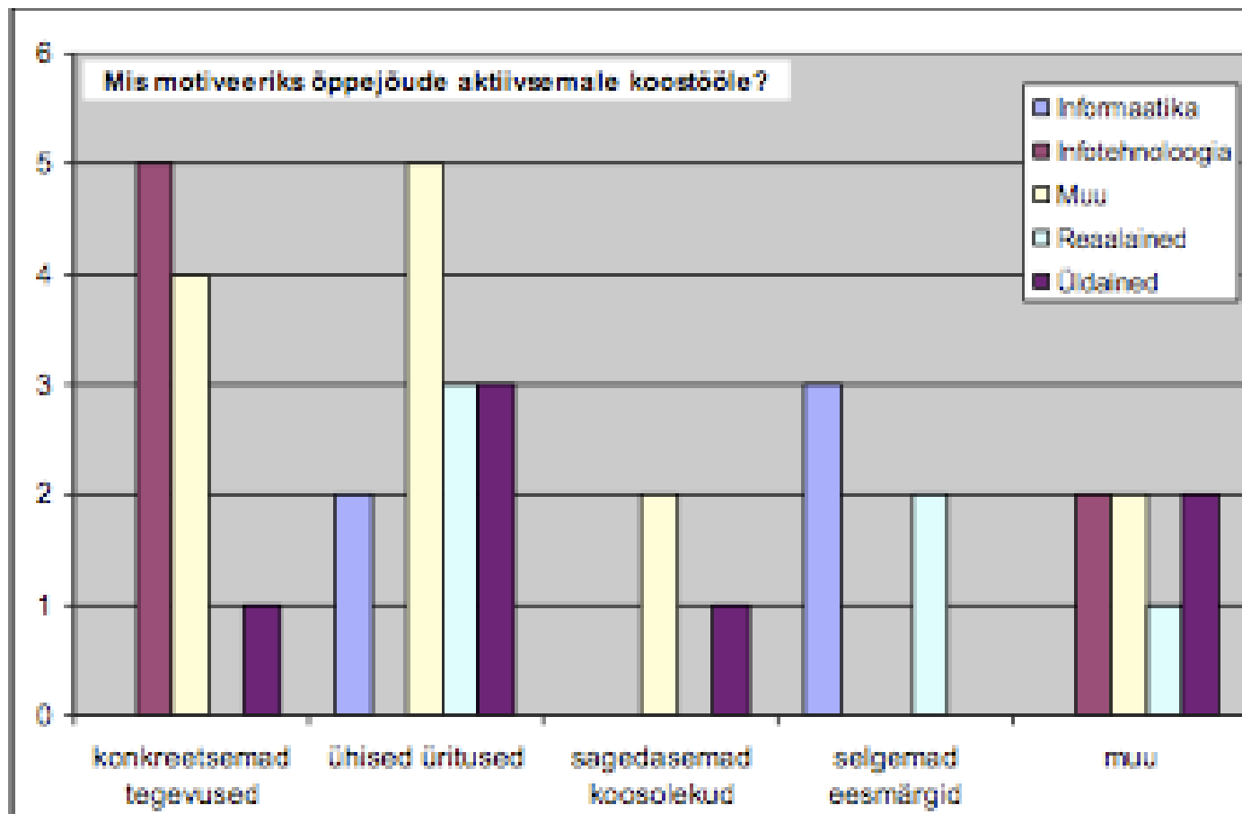
Joonis9: motivatsioon
